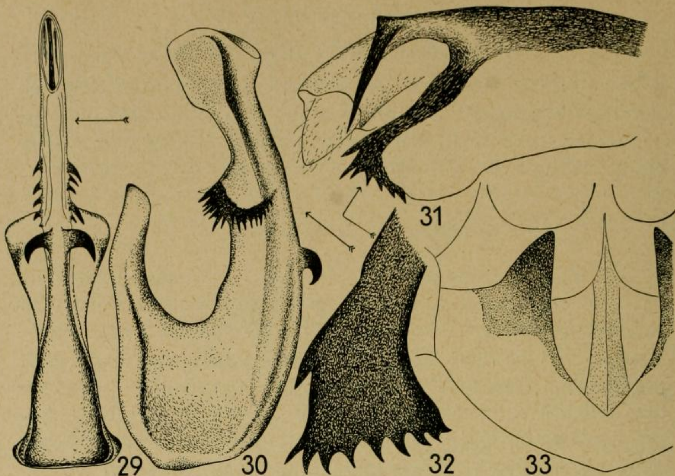
Anoplotettix sahtyiancii sp. n. 29: Aedoeagus von hinten, 30: Aedoeagus von der Seite, 31: Pygophor und Afterröhre von der Seite, 32: Bedornung des Pygophorrandes, 33: VII. Sternit beim Weibchen.
