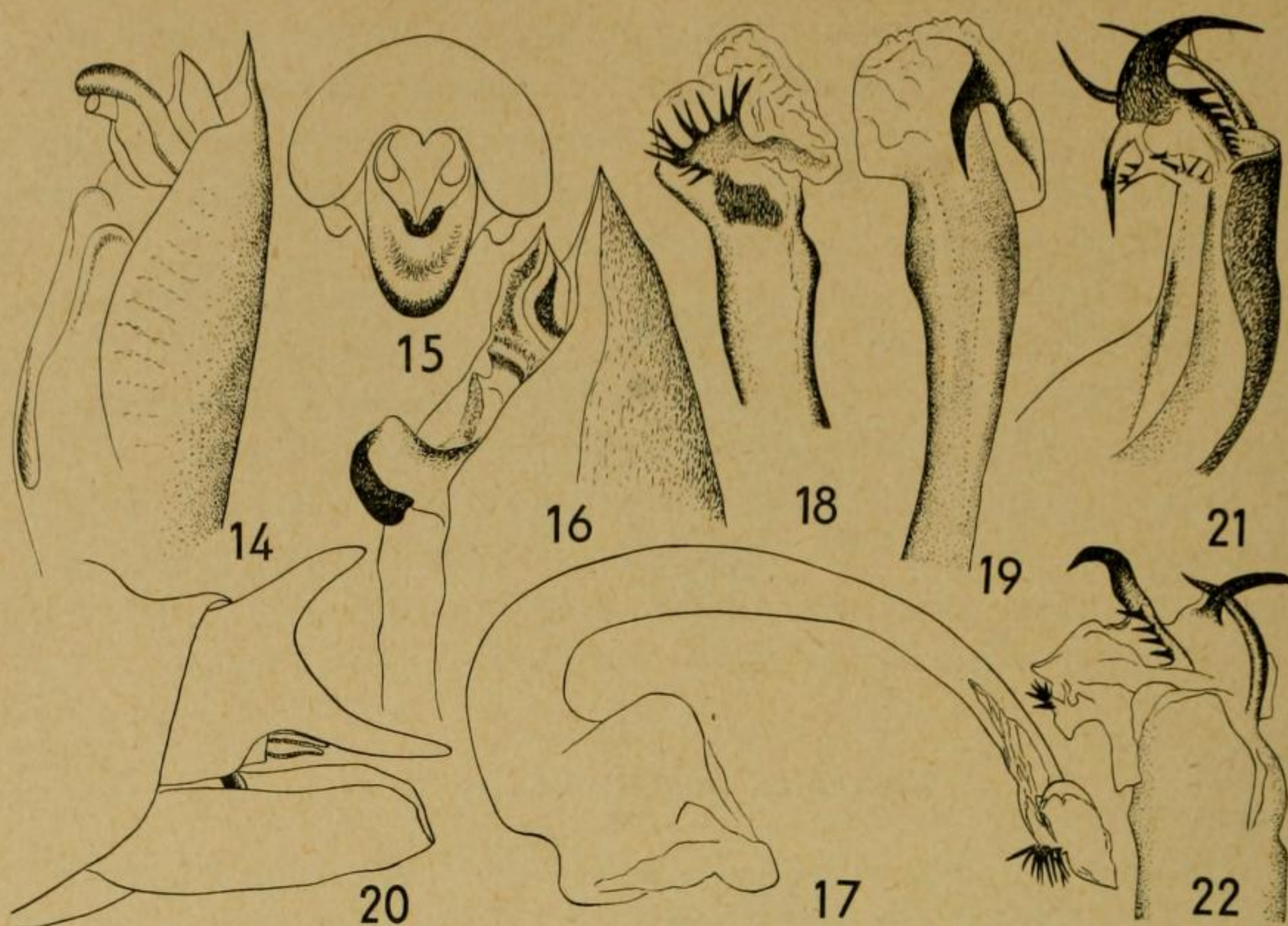
Tibicen esfandiarii sp. n. 14: Genitalblock, 15: Afterröhre und Pygofer von hinten, Cicadatra zahedanica sp. n. 16: Genitalblock-Apex, 17: Aedoeagus von der Seite, 18: Apex am Aedoeagus, ventral, 19: Apex am Aedoeagus von der Seite, 20: Cicadatra kermanica sp. n., 20: Genitalblock von der Seite, Psalmocharias flava sp. n., 21: Aedoeagus-Apex von der Seite, 22: Aedoeagus-Apex ventral.
